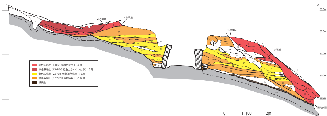
墳丘横断面図 (1 次墳丘と 2 次墳丘がある)
